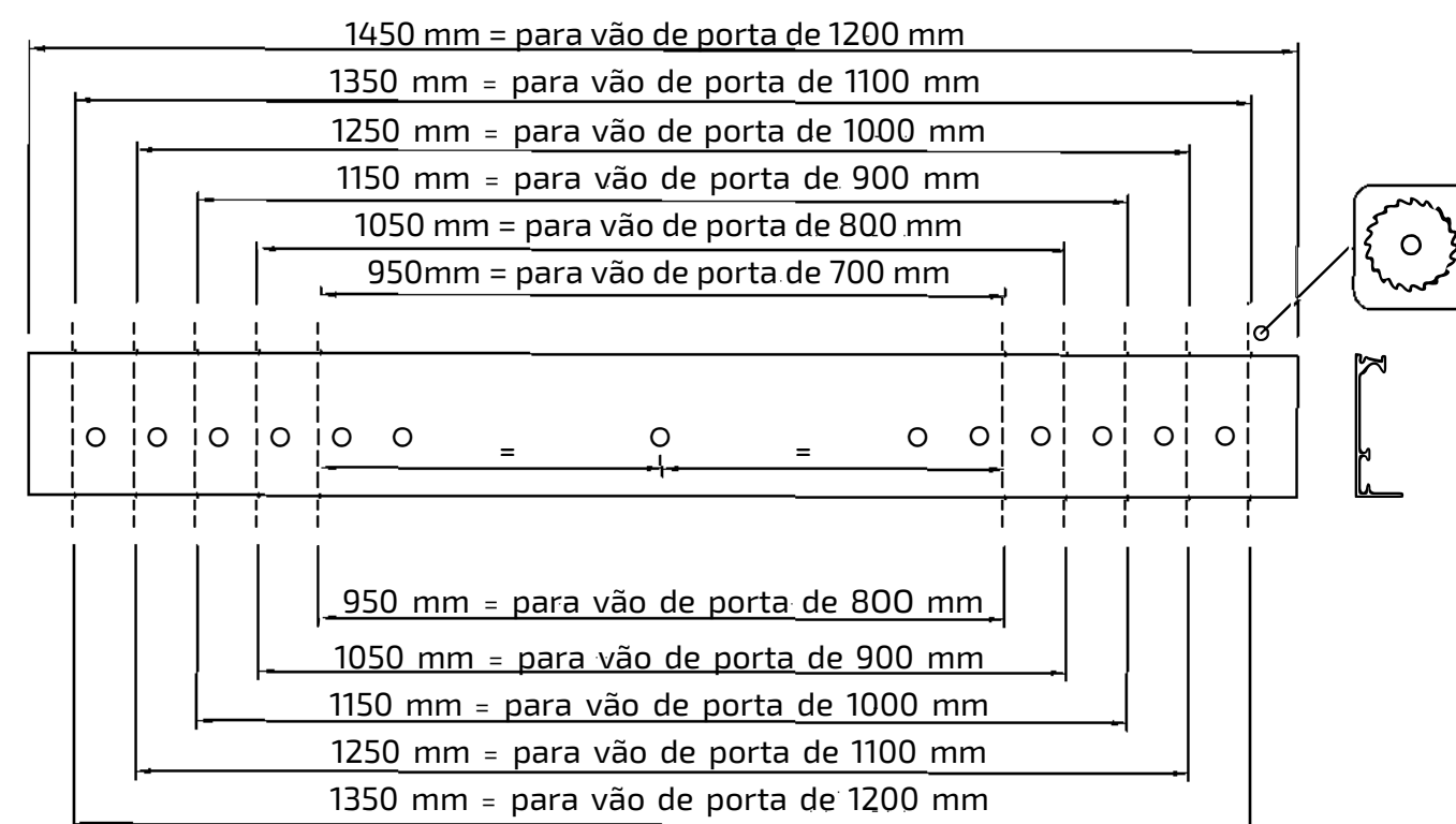
Medidas de corte para montagem simétrica
