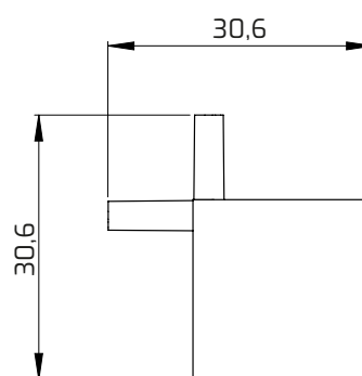
Ângulo 90° externo
