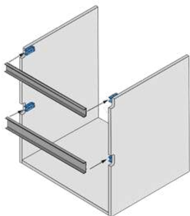
Aplicação horizontal
