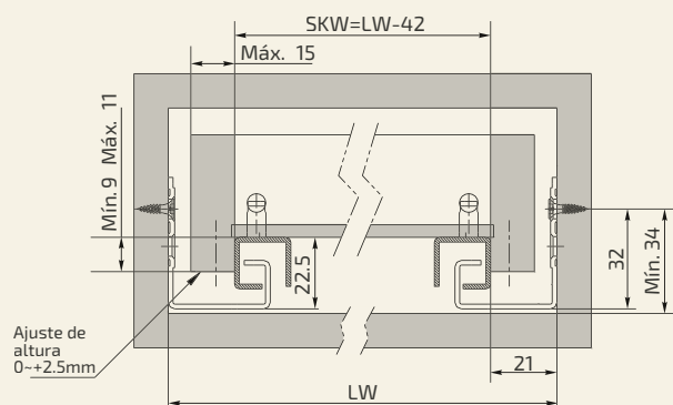
Preparação do Fundo da Gaveta (mm)
