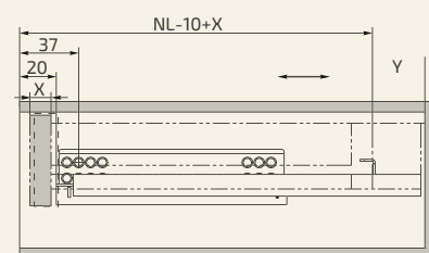
Posições dos Parafusos das Corrediças (mm)
