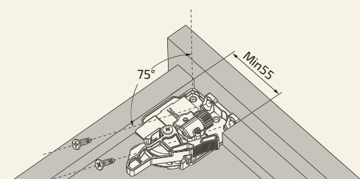
Instalação do Dispositivo de Travamento (mm)
