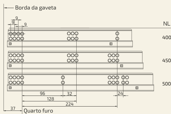
Instalação do Dispositivo de Travamento (mm)
