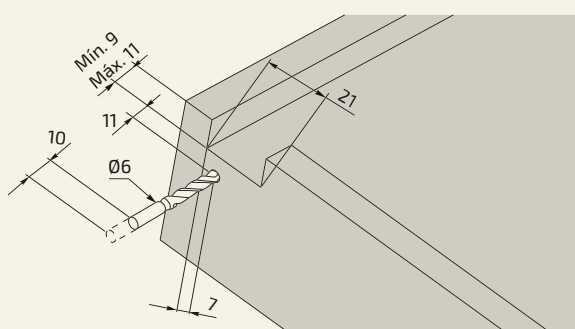
Preparação do Fundo da Gaveta (mm)
